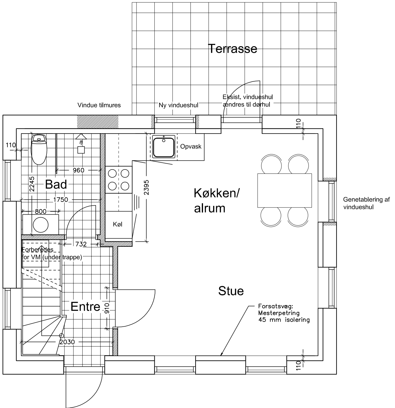
STUEPLAN, MÅL 1:50
